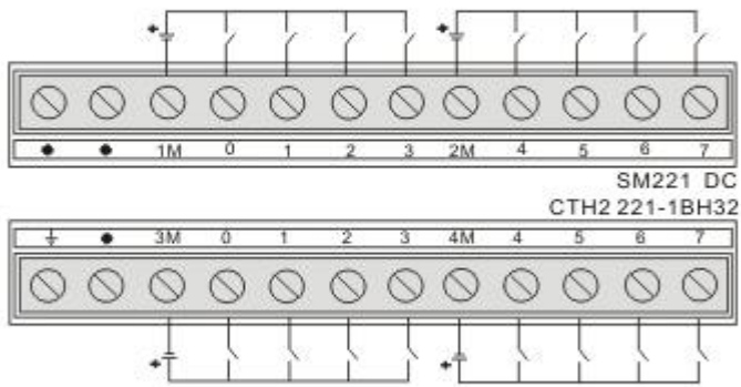
CTH2 221-1BH接线图
