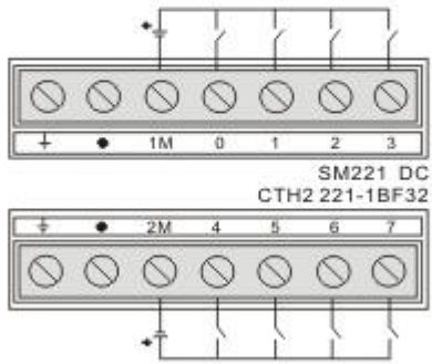
CTH2 221-1BF接线图
