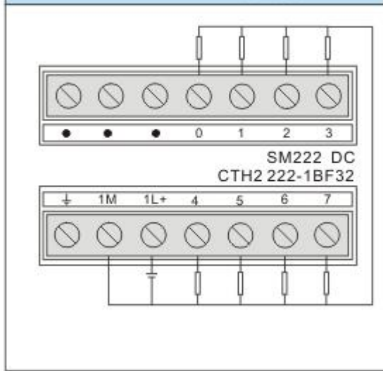
CTH2 222-1BF接线图
