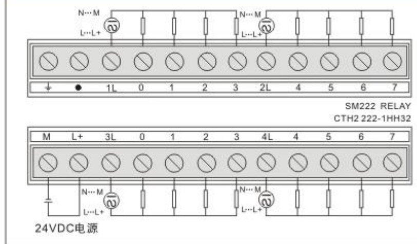
CTH2 222-1HH接线图
