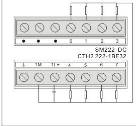
CTH2 222-1BF接线图
